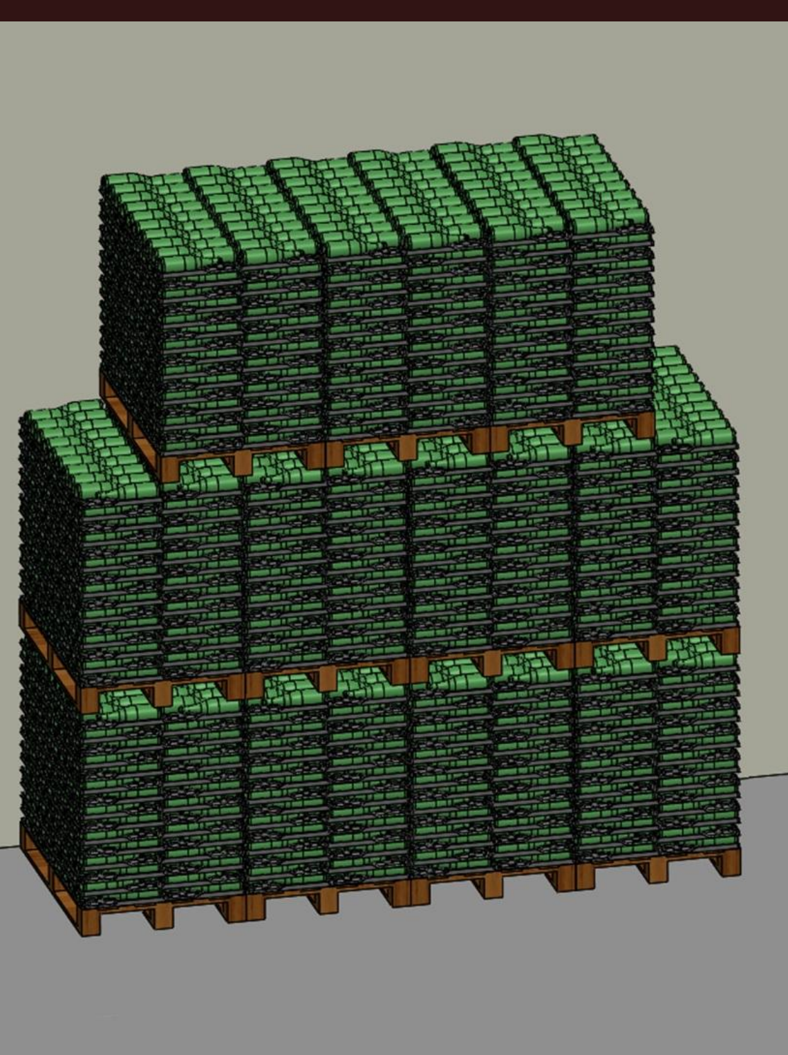
Vinumpro Mod.Nº5 – Botella clásica para vino espumoso, palés de 15 niveles, apilados en 3 palés para un total de 45 niveles. Cada palé contiene 570 botellas.
